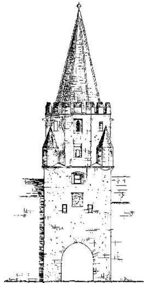
Ansicht von Osten (Stadtseite)
