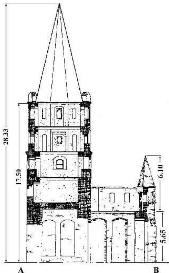
Längsschnitt durch den Torturm und den Vorhof
